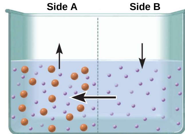
Water Diffusion
