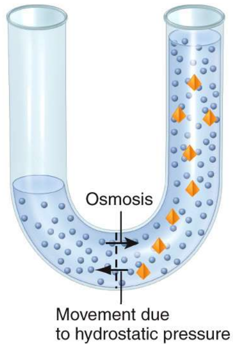
(b) Equilibrium
